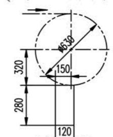
重锤双刮板清扫器安装孔尺寸
